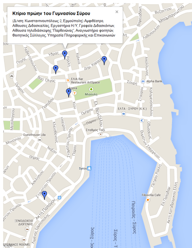
Εικόνα 13. Χάρτης κτιρίων.
